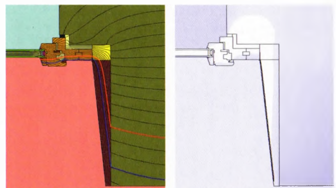
5 Eine keilförmige Innendämmung an der Laibung schafft Abhilfe bei diesem schimmelgefährdeten Anschluss.
