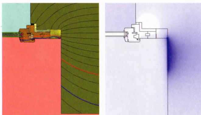
4 Hier zeigt der Versprung des Isothermen-Verlaufs an der Fensterlaibung, wo Schimmel zu erwarten ist. Die Feuchtigkeits-Berechnung weist den Bereich in Dunkelblau aus.
