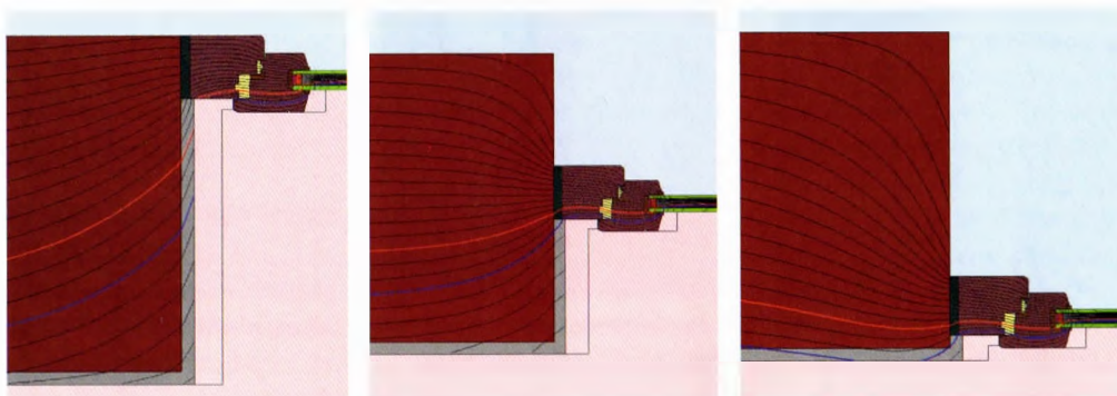
6 Verlauf der 9°C- und 13°C-Isothermen am Wandanschluss bei unterschiedlicher Einbausituation des Fensters (außen bündig (1), mittig (2), innen bündig (3)). Gut zu erkennen: Auch ein sehr weit innen positioniertes Fenster kann eine Wärmebrücke nach sich ziehen.
